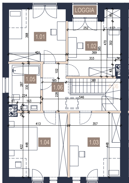
PIĘTRO - 78,62 m 2
